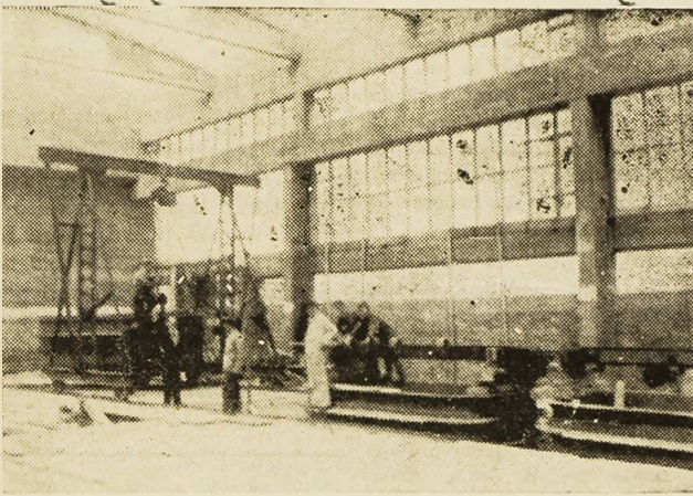
Tvornica i valjaonica aluminija Montaža elektrolitičkih peći
