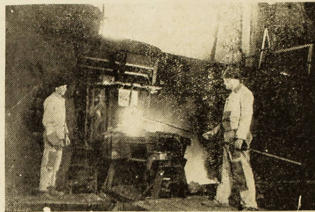
Monofazna peć za proizvodnju fero legura
